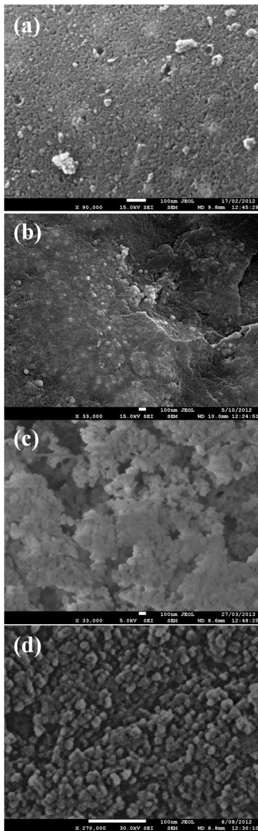
Fig. S2. SEM images of four catalysts (a) CZC-1; (b) CZC-2; (c) CZC-3; (d) CZA
