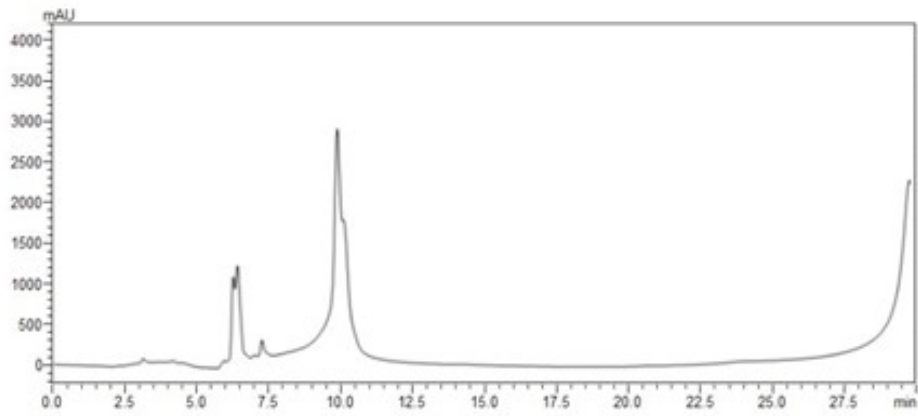
(d) Chromatogram of Cu-2 treated plants
